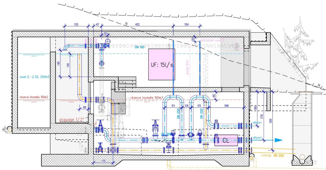
Appareillage du réservoir de Plumachit
